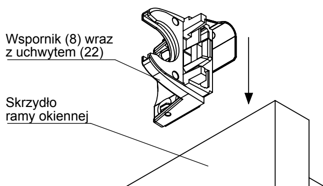
Instalacja górnego uchwytu bezinwazyjnego oraz wspornika na ramie okiennej
