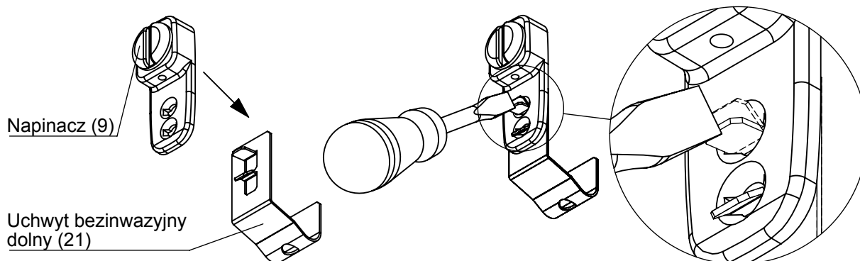
Łączenie dolnego uchwytu bezinwazyjnego oraz napinacza
