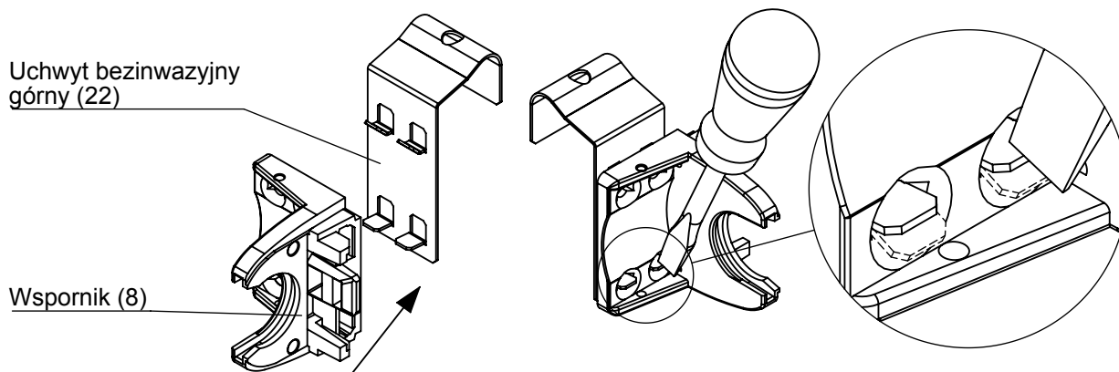
Łączenie górnego uchwytu beziwazyjnego oraz wspornika
